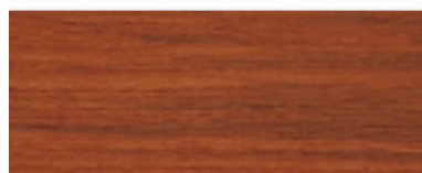
Teak
